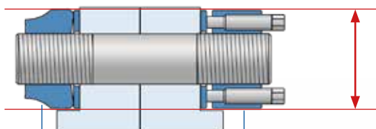
HEICO-TEC® Reactiemoer
